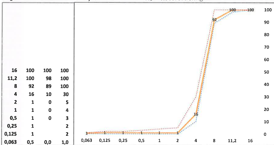
Sigter Forv. Min. Maks DS/EN 933-1 - Kornstørrelsesfordeling
